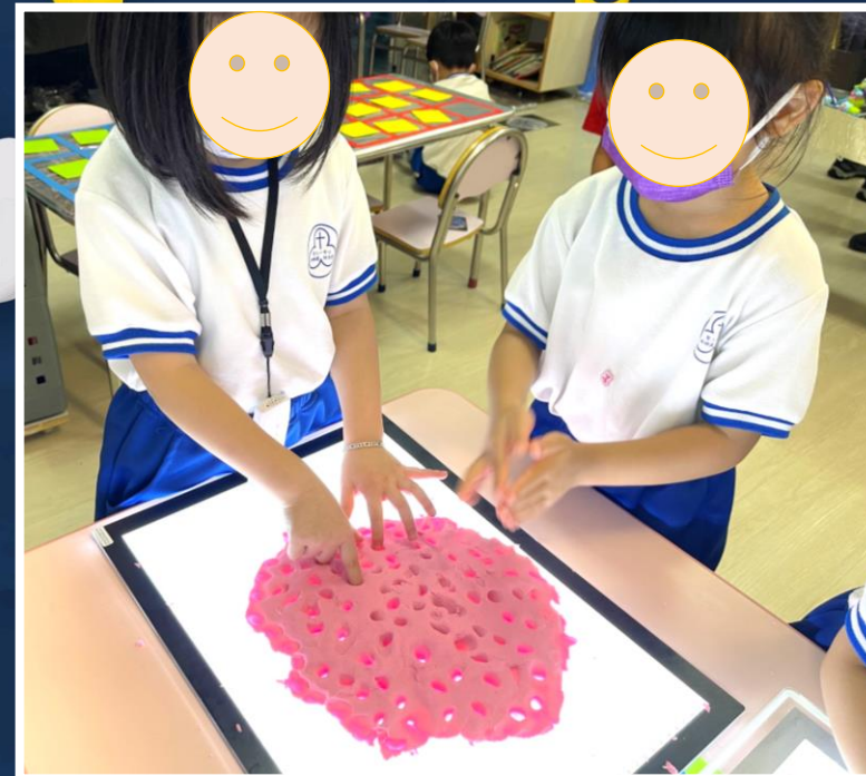
太空岩石
